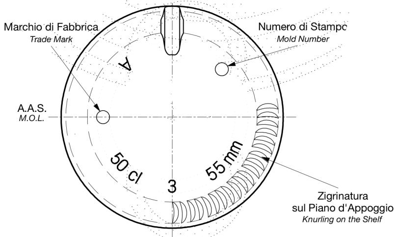
VISTA DAL FONDO Bottom View
