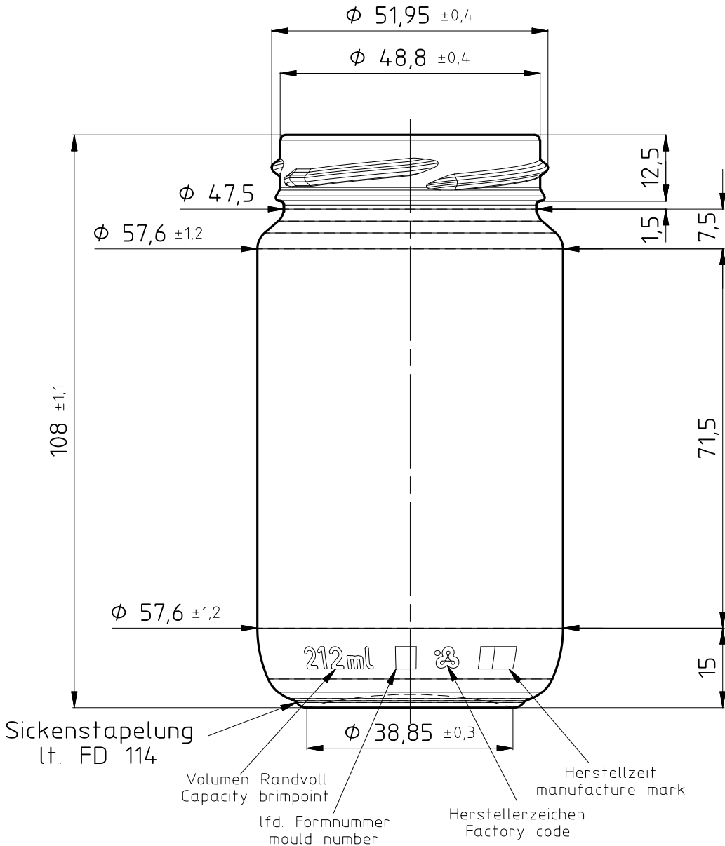
53mm Twist-Off-Mundstück nach EN ISO 9100-6
